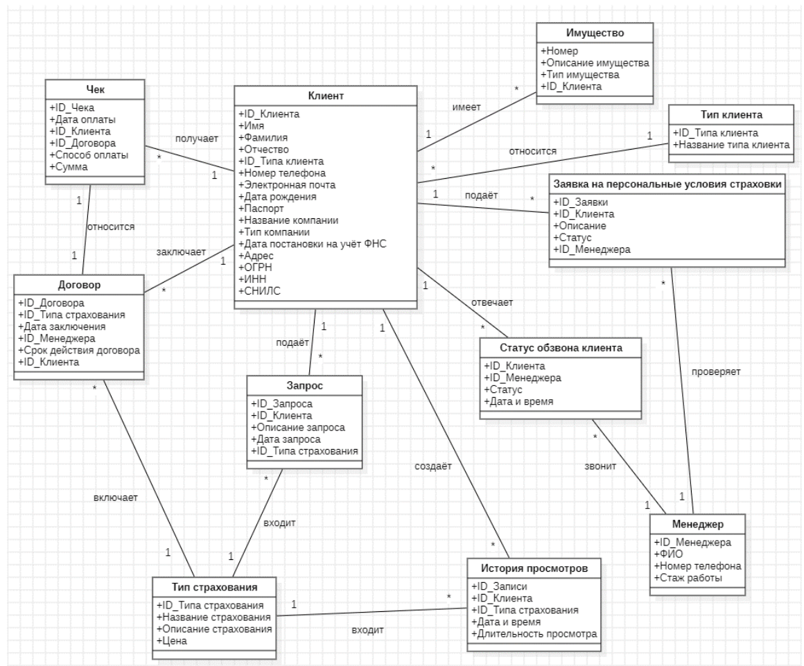
Рисунок 2 – ER-диаграмма
